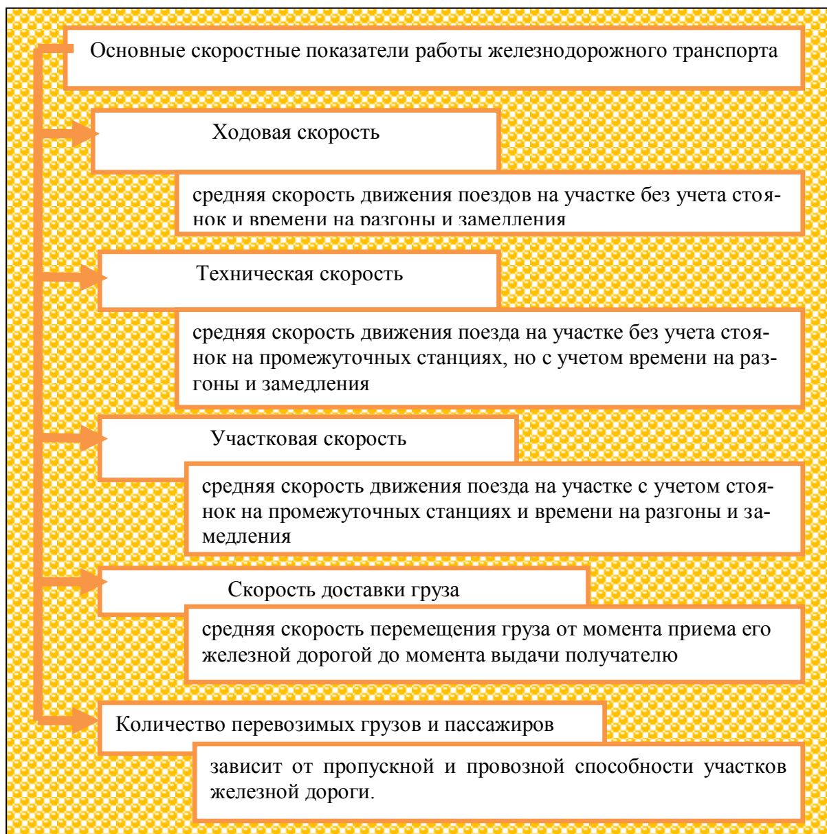
Рисунок 1.5- Основные скоростные показатели работы железнодорожного транспорта
